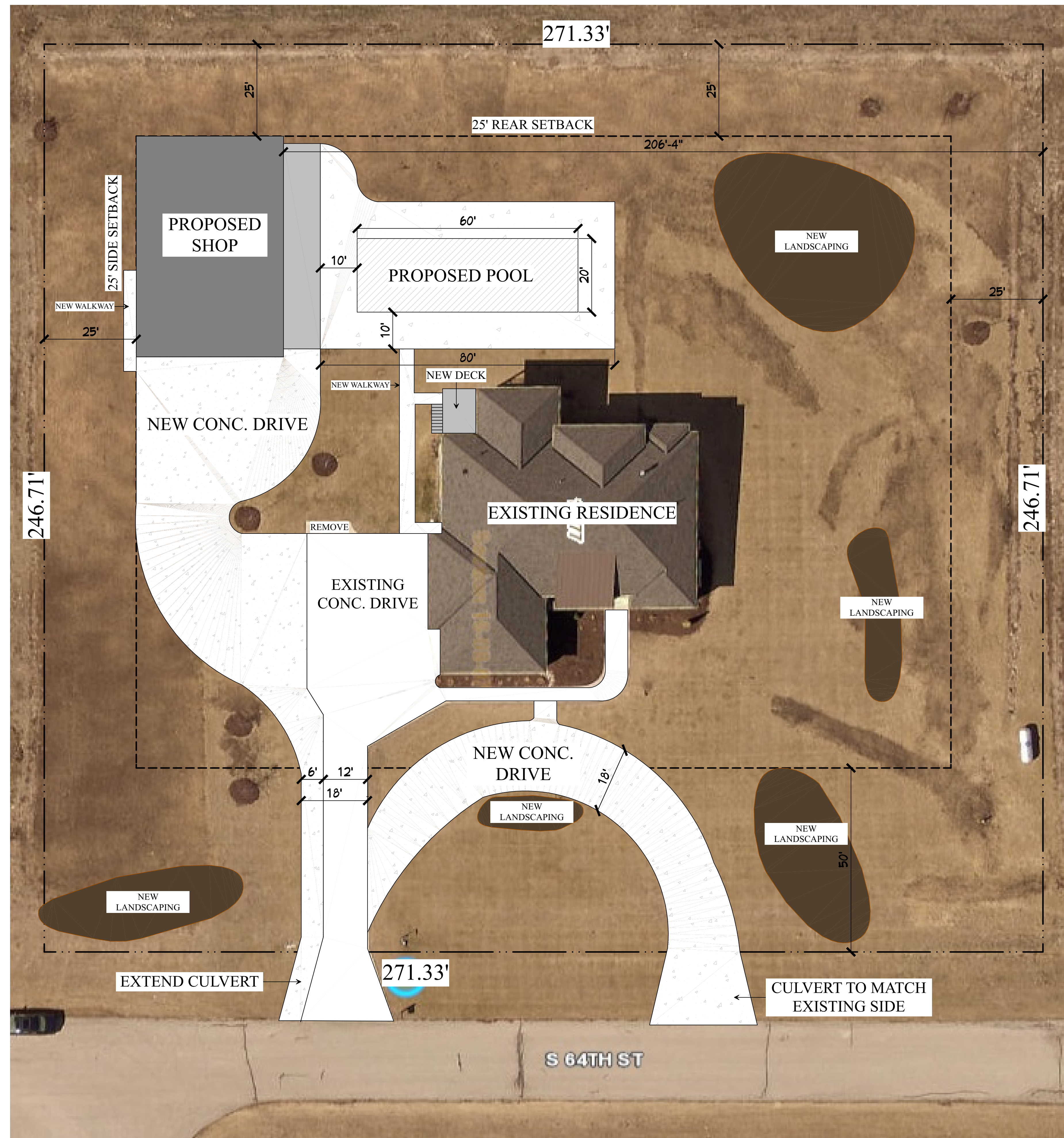
SITE PLAN SCALE: 1" = 15'
